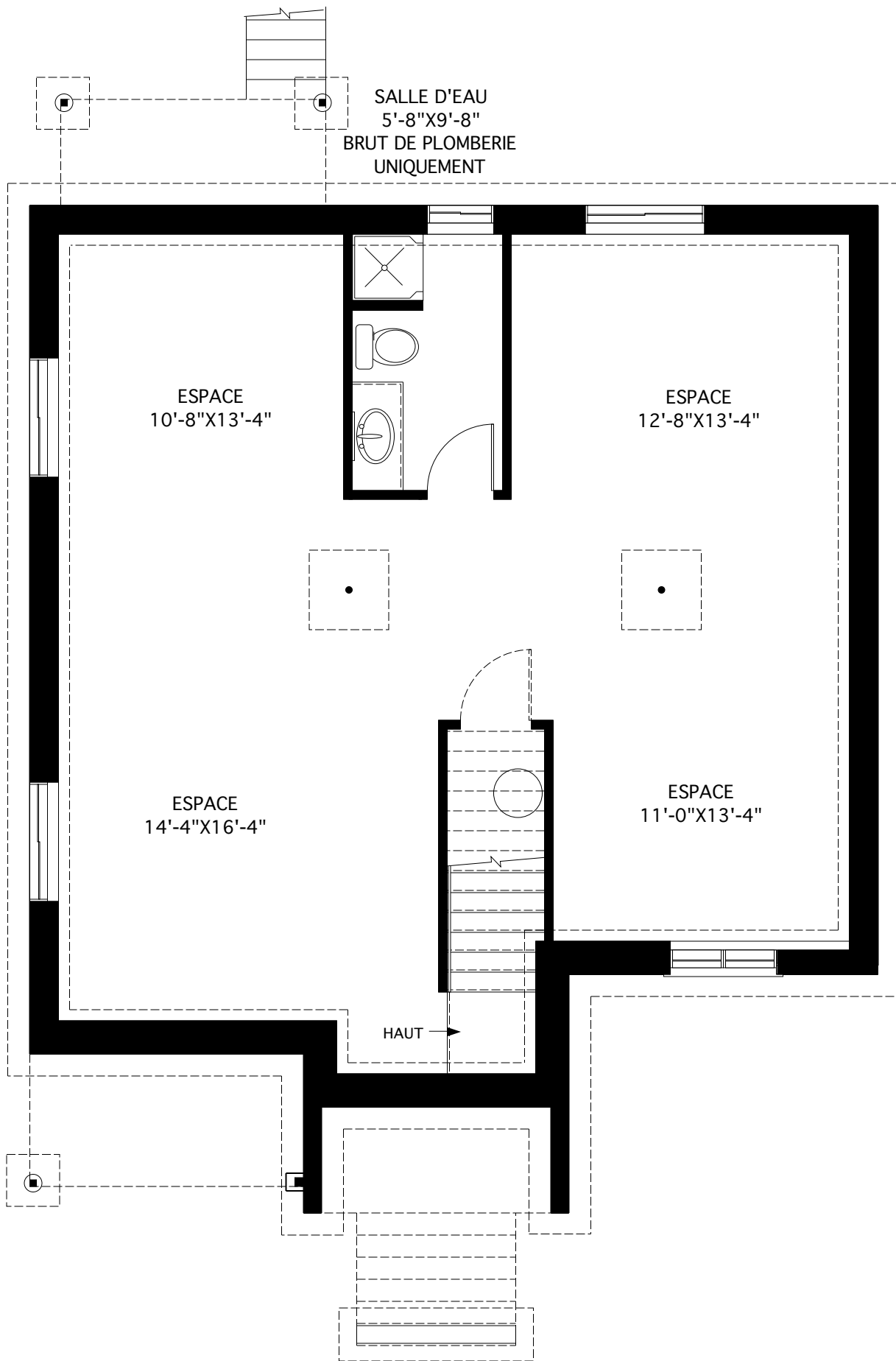
PLAN DU SOUS-SOL SURFACE DE 1,009 pi.ca. (98.77 m.c.)
