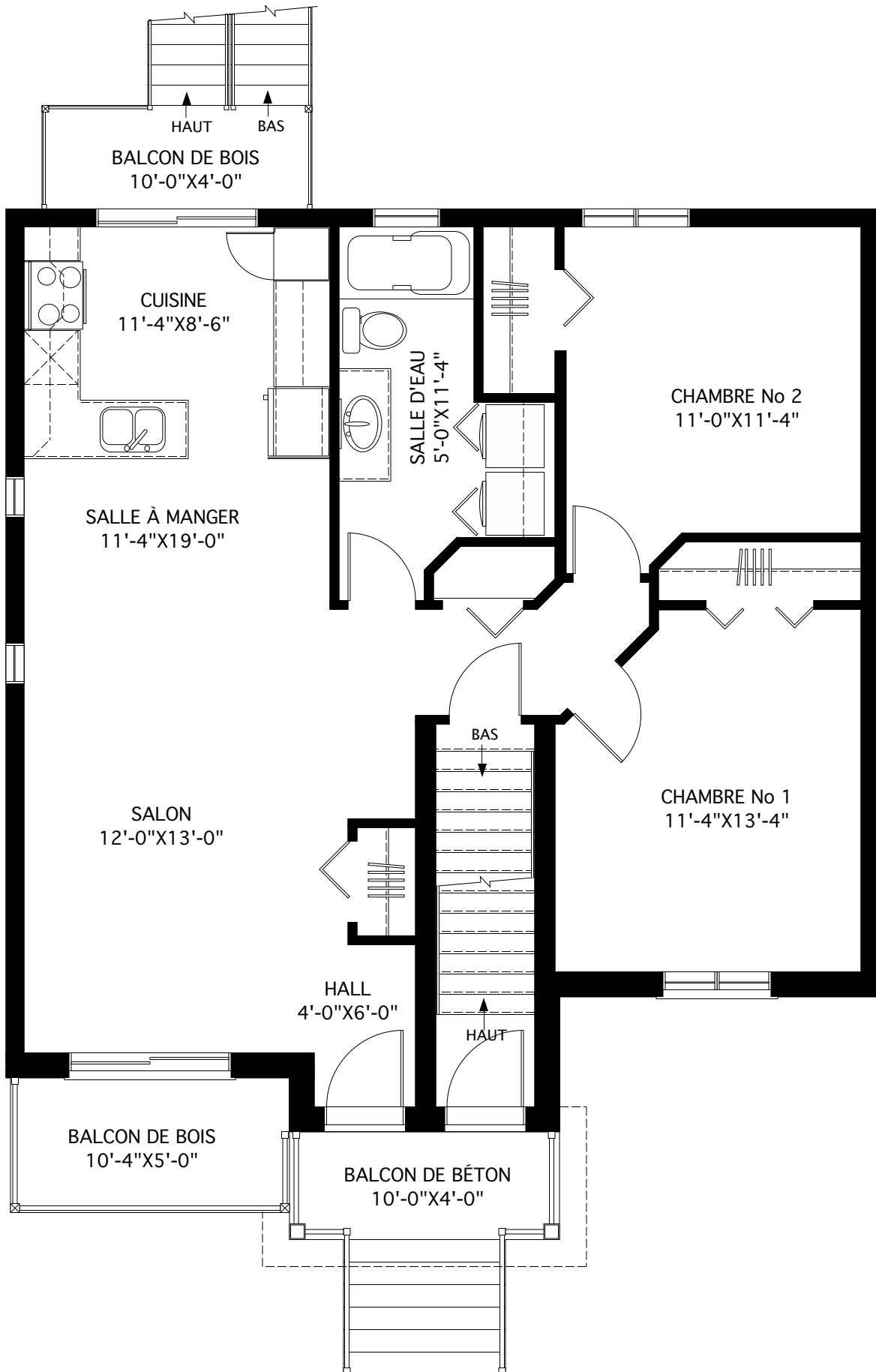
PLAN DU 1 er NIVEAU SURFACE DE 1,009 pi.ca. (98.77 m.c.)
